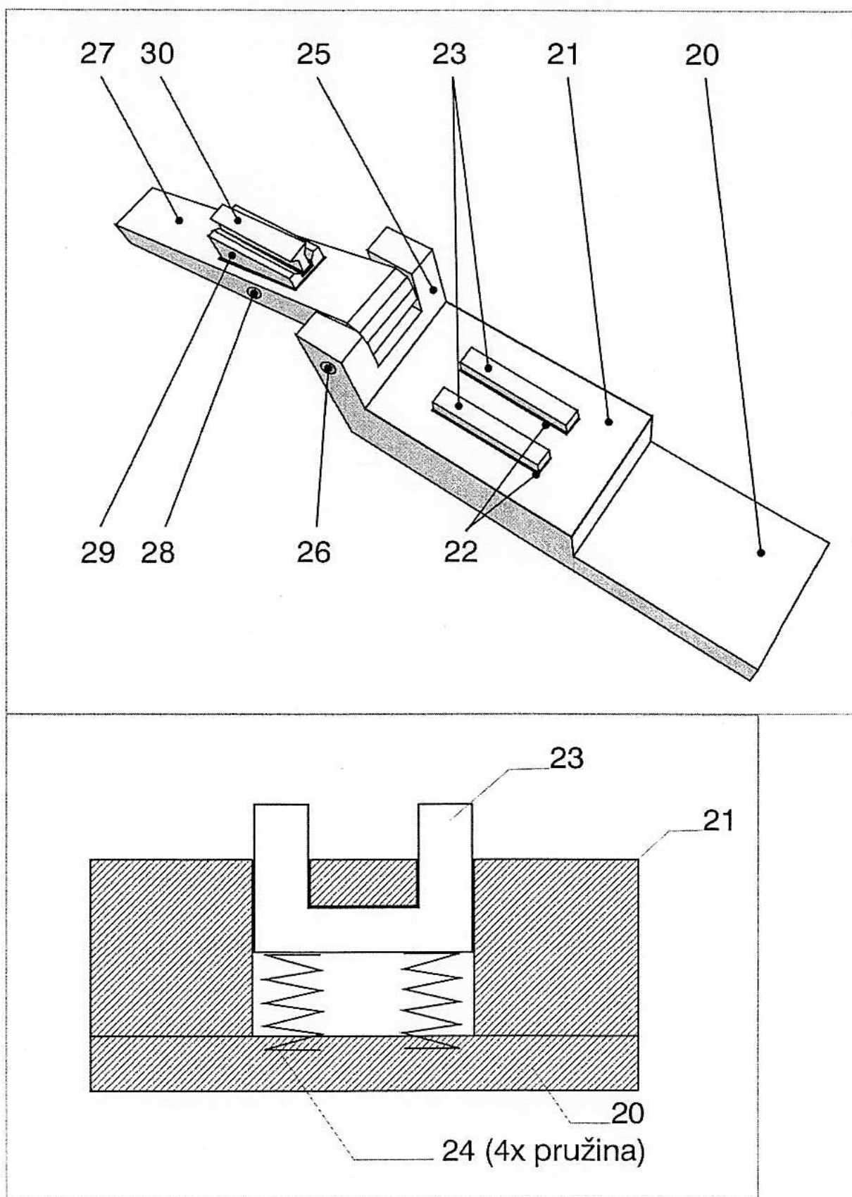
Schéma malého lisovacieho zariadenia.
